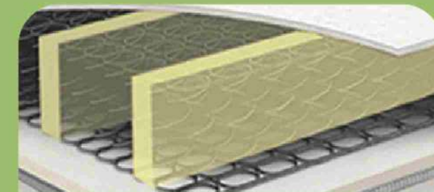
فوم های تیغه ای شکل جهت ساپورت فنر
